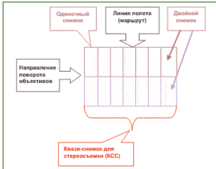
Рис. 2 Схема съемки АФК VisionMap А3
